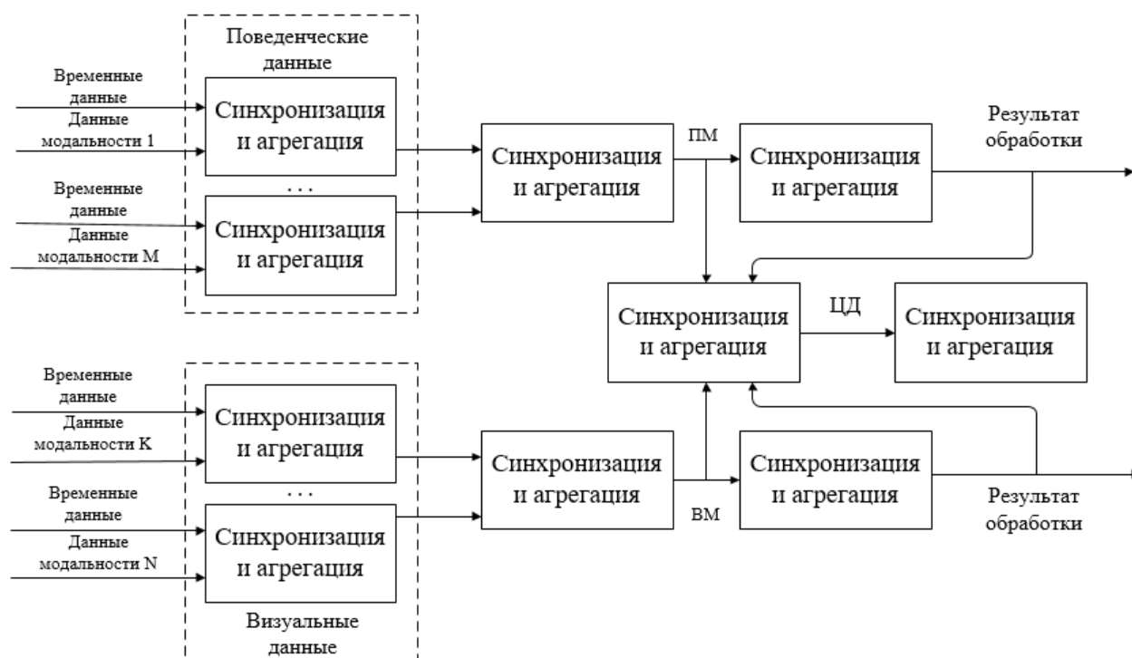
Рис. 3. Схема модели исчисления для цифровых двойников
