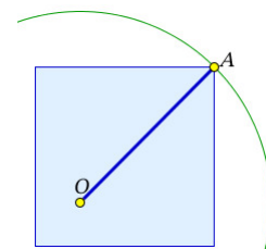
Рис. 1. Нахождение \sup(A)
